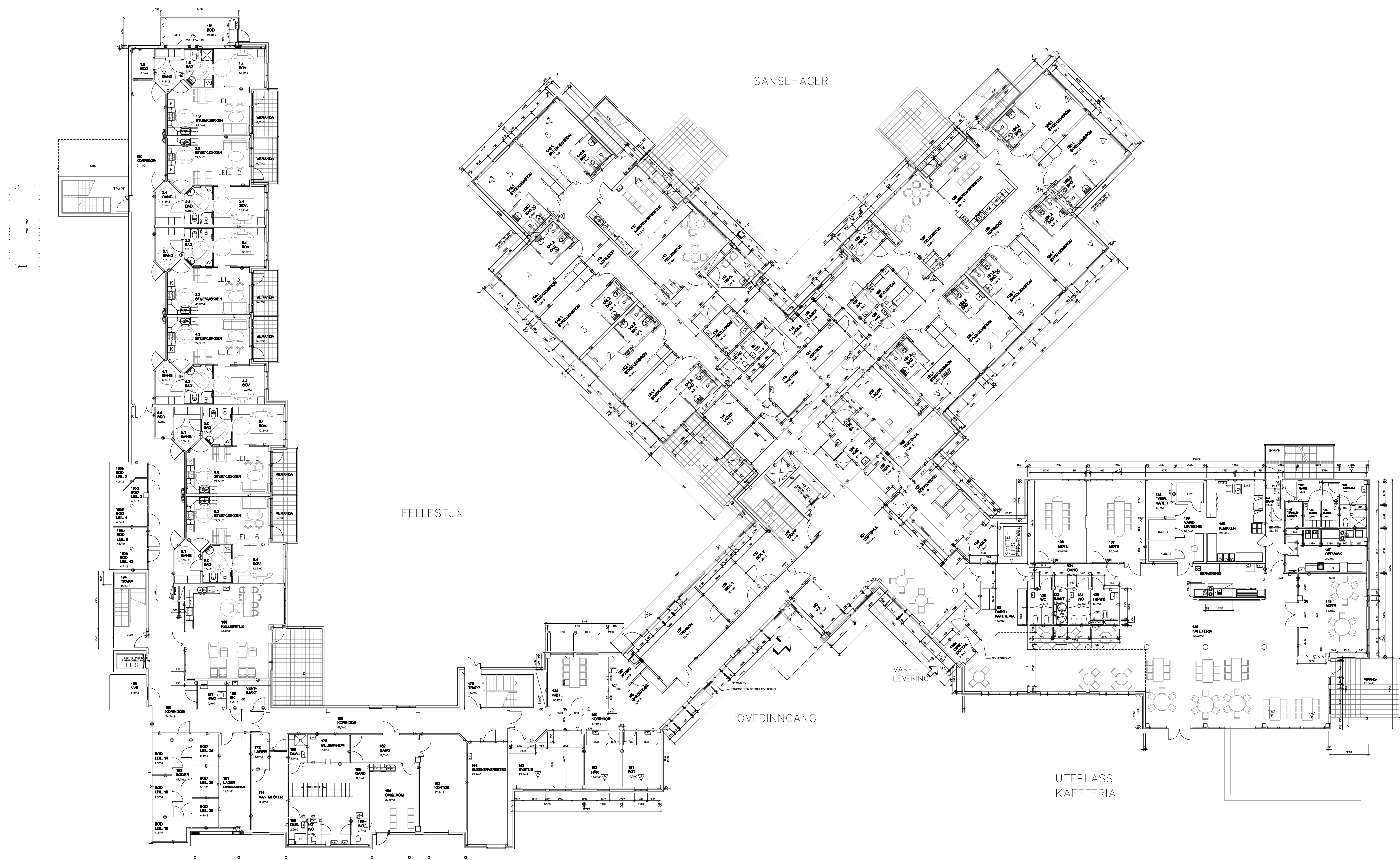
PLAN 1. ETG.
